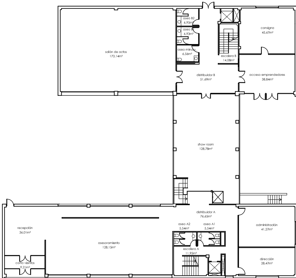
PLANTA BAJA (1/300)
