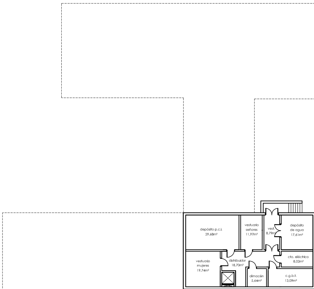
PLANTA SÓTANO (1/300)
